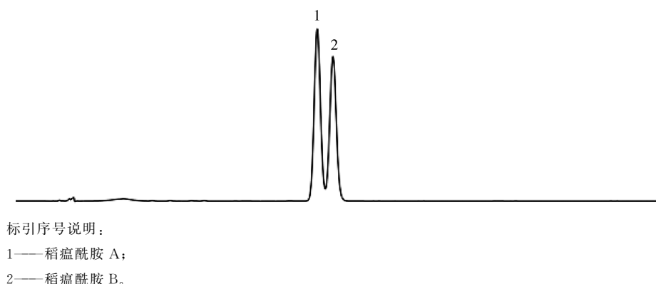
图 1 稻瘟酰胺悬浮剂的高效液相色谱图
