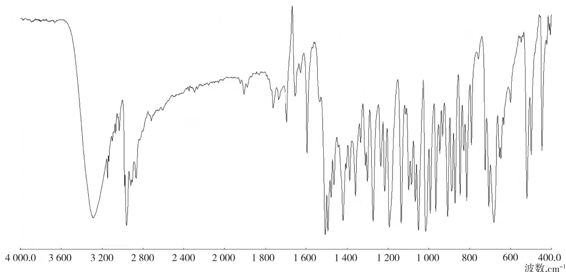
图 1 烯效唑标样的红外光谱图
