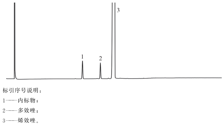
图3 烯效唑原药与内标物的气相色谱图(测定多效唑)
