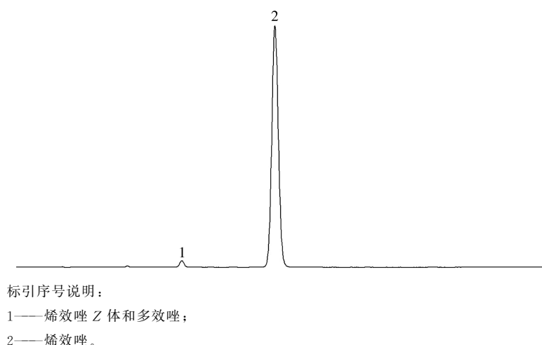
图 2 烯效唑原药的高效液相色谱图
