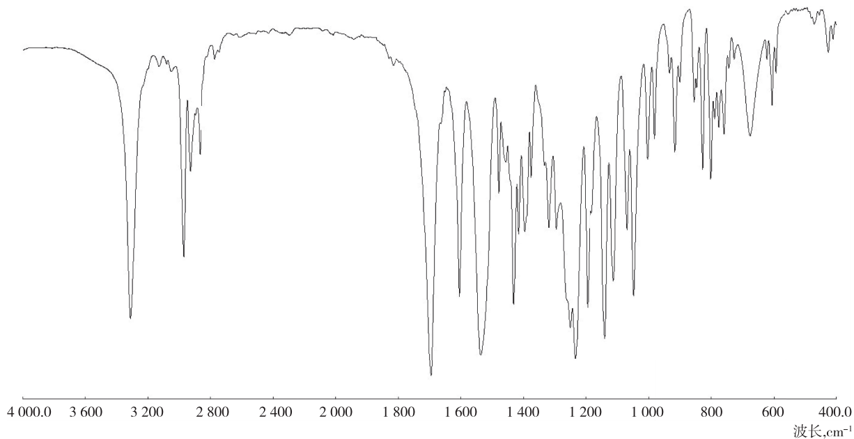
图 1 乙霉威标样的红外光谱图
