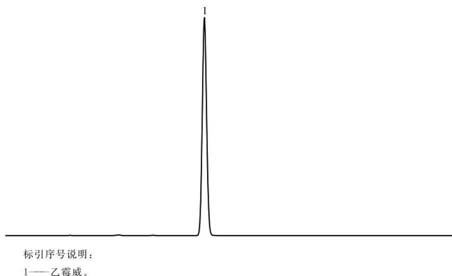
图2 乙霉威原药的高效液相色谱图
